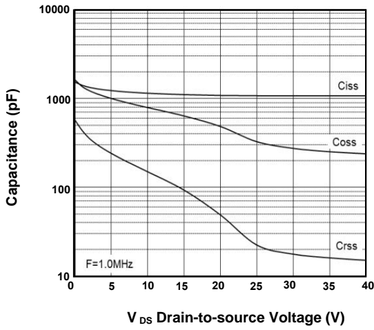
FIG.7- Capacitance
